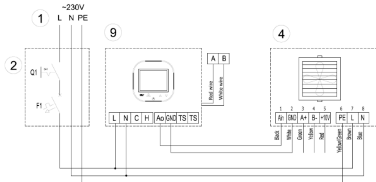
Przykładowy schemat podłączenia nagrzewnicy Volcano EC, pełne schematy elektryczne dostępne do pobrania na www.vtsgroup.com Example connection diagram of Volcano EC, full electrical diagrams available for download at www.vtsgroup.com .
